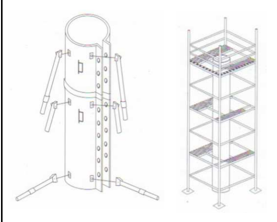
Coffrer
